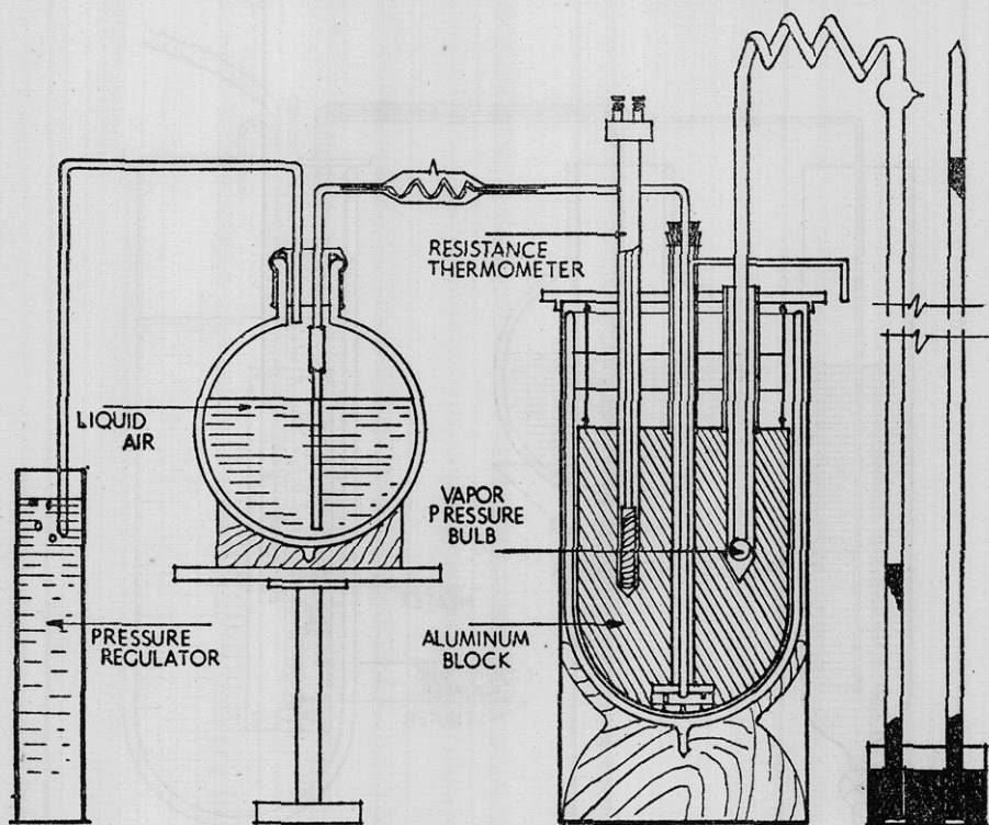
FIG. 5. Type e cryostat
